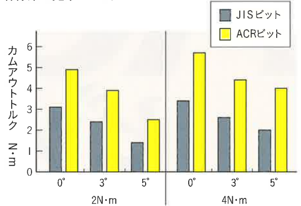
ビット挿入時の傾きと推力
